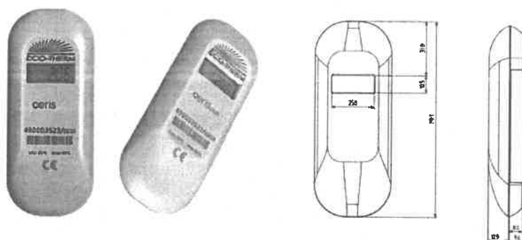
Fot. Podzielnik kosztów ogrzewania Ceris firmy APATOR
