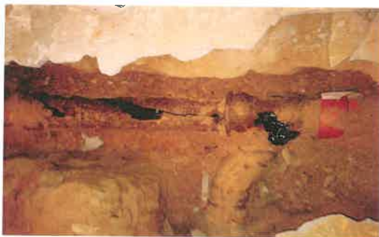
Fot. Fragment starej uszkodzonej rury kanalizacji poziomej w piwnicy budynku Siemiatycka 1 klatka 1.
